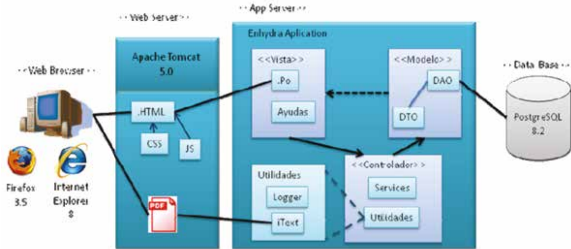
Figura 3. Arquitectura de SIRESS
