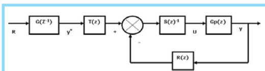
Figura 3. Esquema del controlador digital RST.
