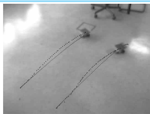
Figura 11. Posición y trayectorias más suaves de los dos robots en la imagen.
