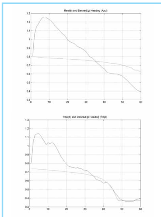
Figura 12. Orientación real del robot azul y rojo en comparación con sus referencias, nótese que el sobre-impulso es menor que en la Figura No. 10.
