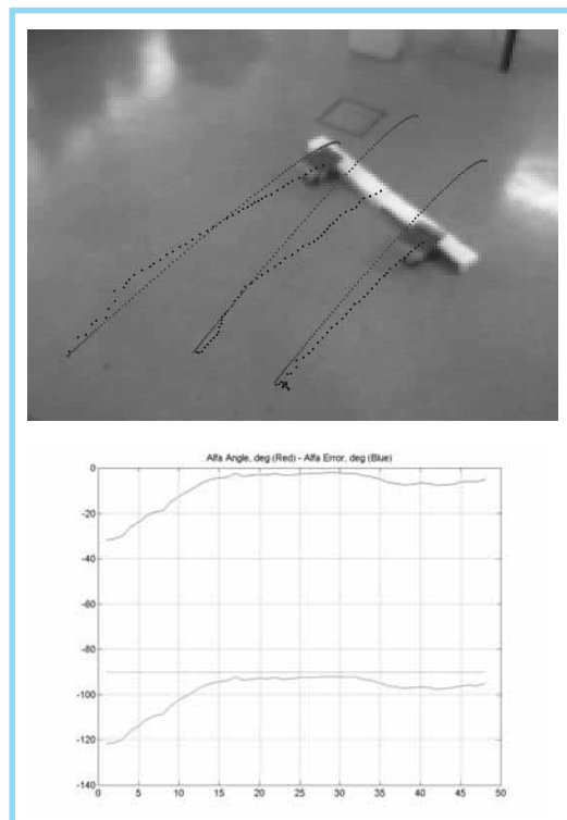
Figura 13. Trayectorias de los robots y la barra en la imagen con una inclinación inicial de la barra mayor a 90^\circ (a); error en la inclinación de la barra (curva superior), orientación de la barra (curva inferior) y referencia (línea constante) (b).
