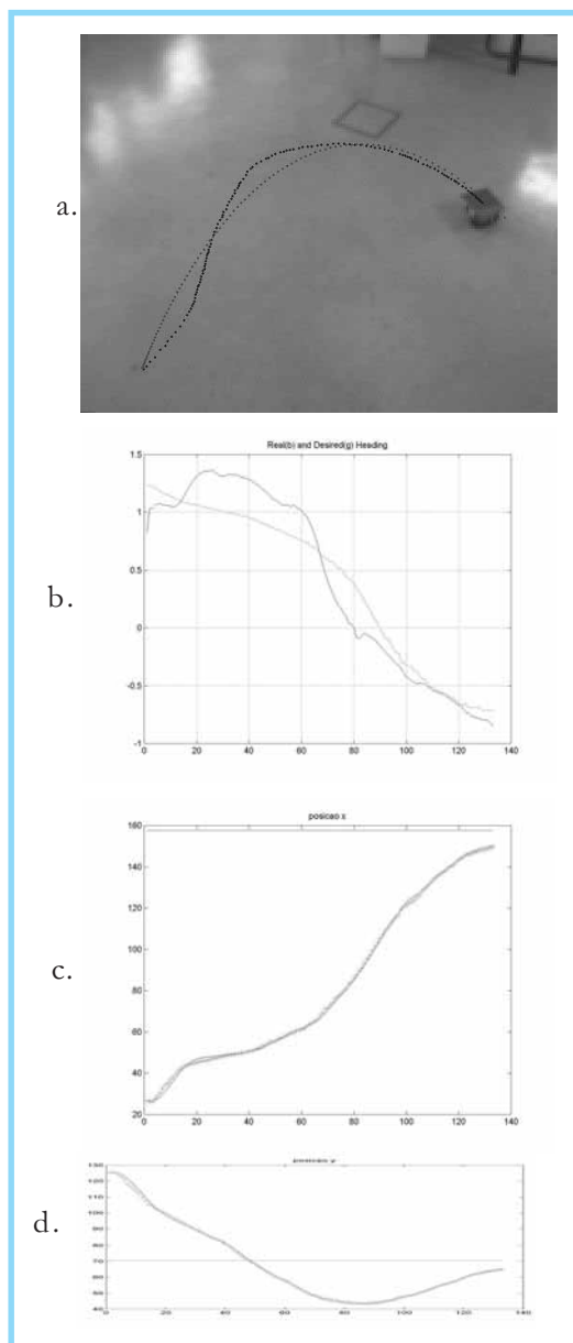
Figura 7. Evolución de la posición del robot azul en una trayectoria curva (a); la orientación del robot y la referencia (línea más suave de la figura) (b); la posición XY del robot (c y d).
