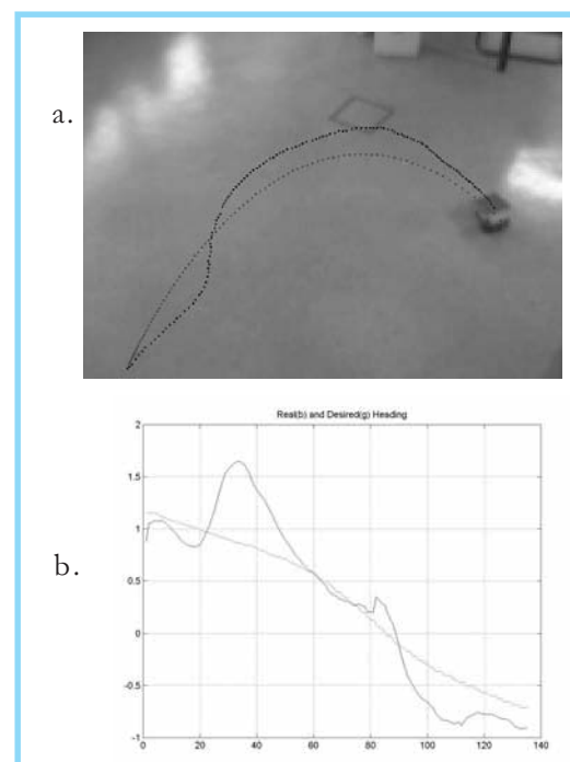
Figura 8. Evolución de la posición del robot rojo en una trayectoria curva (a); la orientación del robot y la referencia (línea más suave de la figura) (b).
