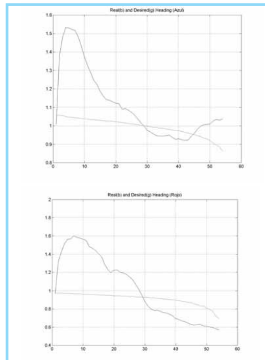
Figura 10. Orientación real del robot azul y rojo en comparación con sus referencias.
