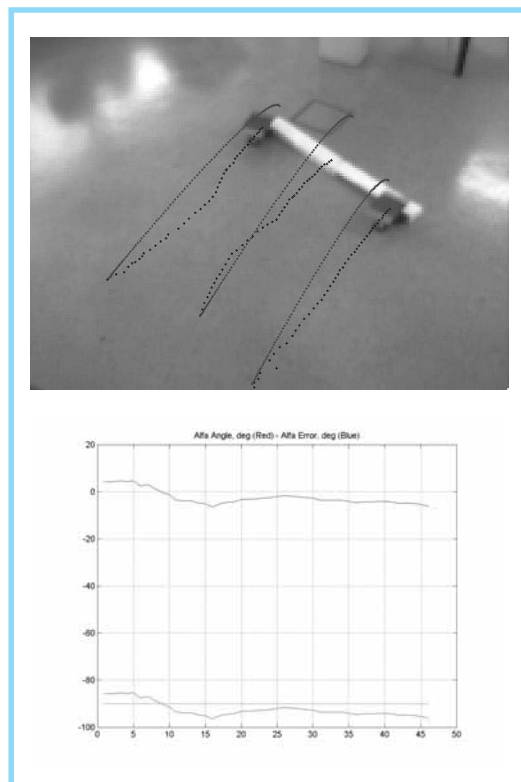
Figura 14. Trayectorias de los robots y la barra en la imagen con una inclinación inicial de la barra menor a 90^\circ (a); error en la inclinación de la barra (superior), orientación de la barra (inferior) y referencia (línea constante) (b).
