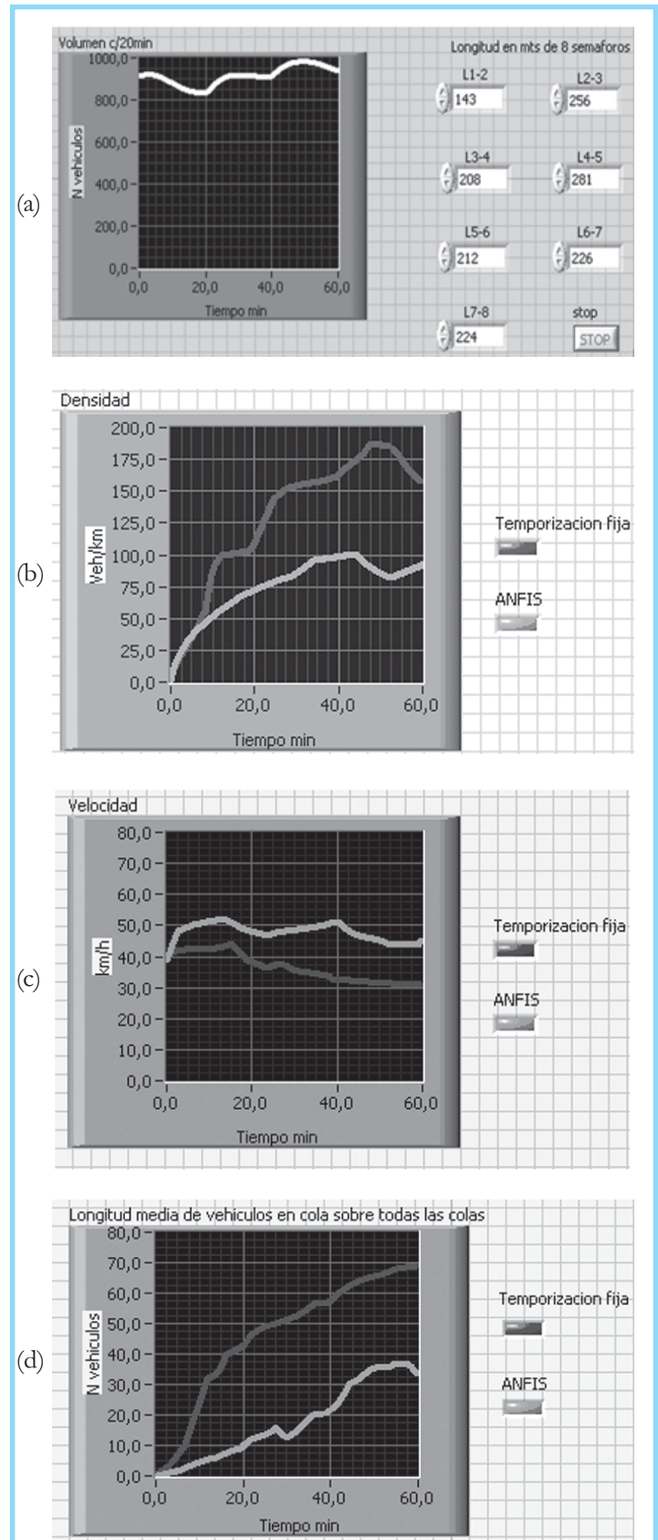
Figura 8. Comparación macroscópica del modelo ANFIS con el modelo de temporización fija. a) Volumen vehicular para periodos de 20 minutos a través de una hora. b) Densidad vehicular en veh/km. c) Velocidad promedio vehicular en km/h. d) Numero promedio de vehículos en cola sobre todas las colas.
