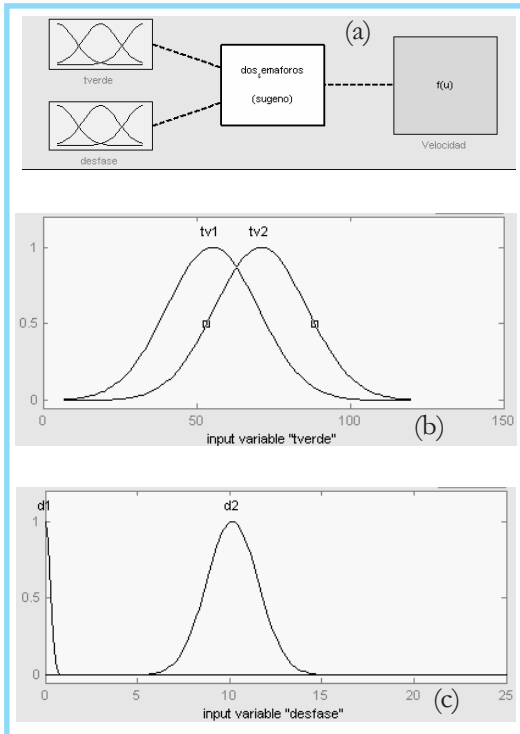
Figura 5. Universos para el sistema ANFIS. a) Universos ANFIS basado en el modelo Takagi-Sugeno. b) Conjuntos gaussianos del universo t_v . c) Conjuntos gaussianos del universo desfase.
