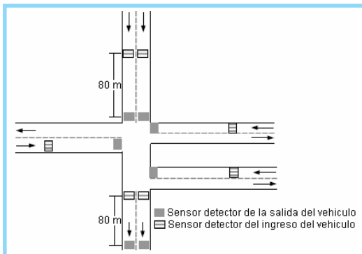
Figura 3. Ubicación de los sensores en la avenida.
