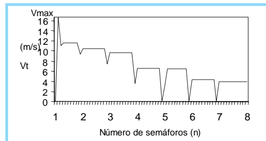
Figura 6. Velocidad promedio de 40 vehículos a través de 8 semáforos de tiempos fijos.
