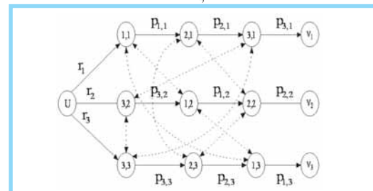
Figura 1. Representación en grafo de un JSSP minimizando tardanza ponderada total en el caso de tres máquinas y tres trabajos [8].
