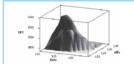
Figura 2. Superficie de respuesta (TPT) en función de los exponentes a (Alfa) y b (Beta).
