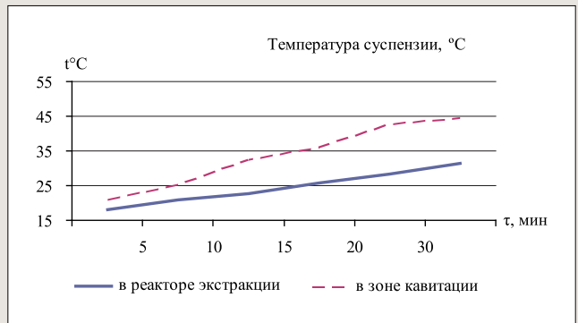
Рис. 2. Зависимость температуры суспензии торфа от продолжительности процесса кавитации
