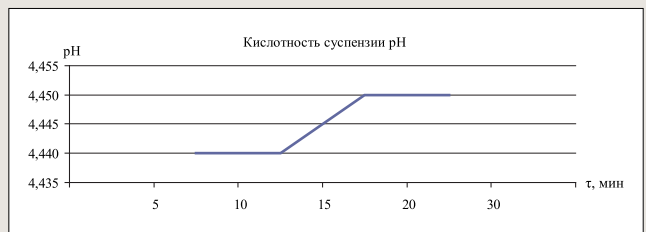
Рис. 3. Зависимость уровня кислотности гуминовых удобрений от времени воздействия кавитации на суспензию торфа
