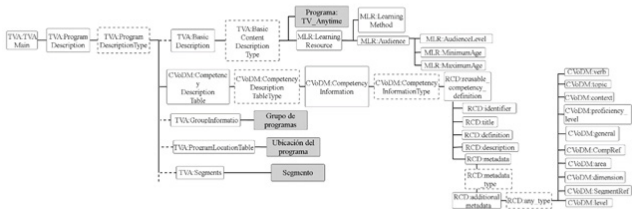
Figura 2. Esquema de metadatos CVoDM.
