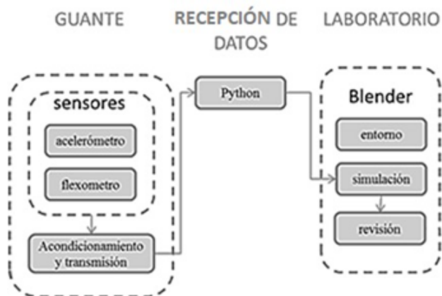
Figura 1: Diagrama de bloques del laboratorio virtual de química para realizar la práctica de metales alcalinos.
