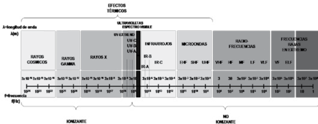
Figura 1. Espectro electromagnético
