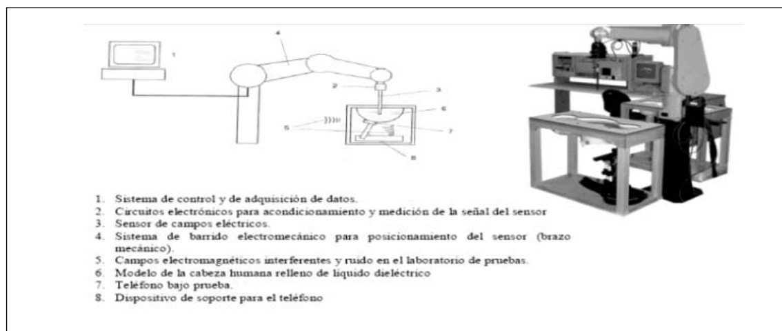
Figura 1. Sistema de medida completo para SAR [5]
