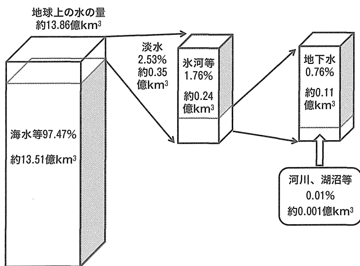
図1 地球上に存在する水の量
