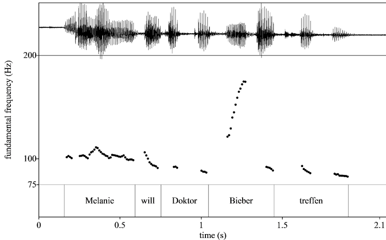
Abbildung 6.8: Screenshot mit (von oben nach unten) Oszillogramm und F0-Verlauf für die Äußerung <Melanie will Dr. Bieber treffen> von Sprecherin M1. Das Zielwort <BIEber> ist im engen Fokus und der nukleare Tonakzent als L+H* klassifiziert.
