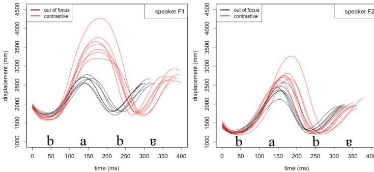
Abbildung 6.20: Trajektorien der Zwischenlippedistanz für Sprecherin F1 (Änderungen im Überlappingsgrad der transvokalischen Öffnungs- und Schließgesten mit zusätzlicher Targetmodifikation) und F2 (Änderungen im Überlappingsgrad der transvokalischen Öffnungs- und Schließgesten ohne zusätzliche Targetmodifikation) verdeutlichen die sprecherspezifische Variation; kontrastiver Fokus versus Hintergrund (out of focus).
