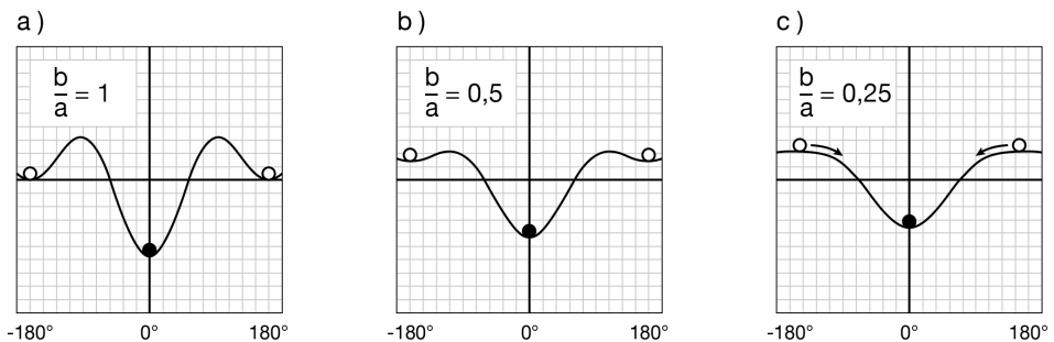
Abbildung 3.1: Potentiellandschaften für unterschiedliche Werte von b/a . Die schwarze gefüllte Kugel markiert die Startbedingung für den In-Phase-Modus, die beiden ungefüllten Kugeln die für die Anti-Phase. Der Attraktor für die Anti-Phase wird in (b) schwächer und verschwindet schließlich in (c). Die Pfeile in (c) markieren den abrupten Wechsel vom Anti-Phase- zum In-Phase-Modus.
