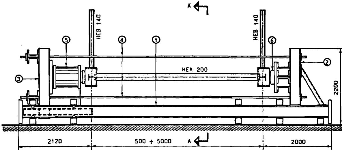
FIG. 1.- HORIZONTAL TESTRIG FOR BEAM-COLUMN SUB-ASSEMBLAGE
