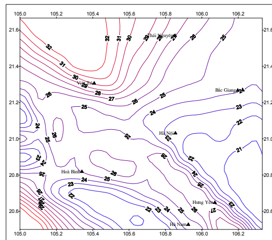
Hình 10. Độ sâu mặt Moho khu vực Hà Nội và kế cận
