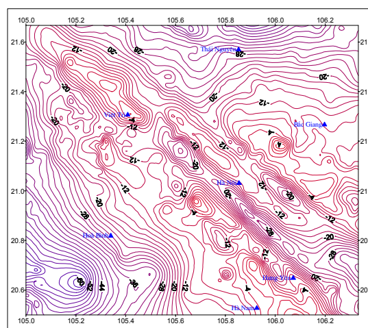
Hình 1. Dị thường trọng lực Bouguer khu vực Hà Nội và kể cận
