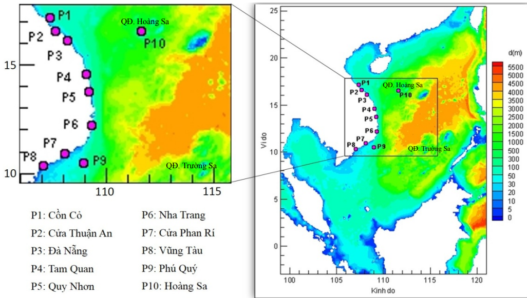
Hình 1. Sơ đồ địa hình khu vực nghiên cứu và vị trí các điểm nghiệm triều
