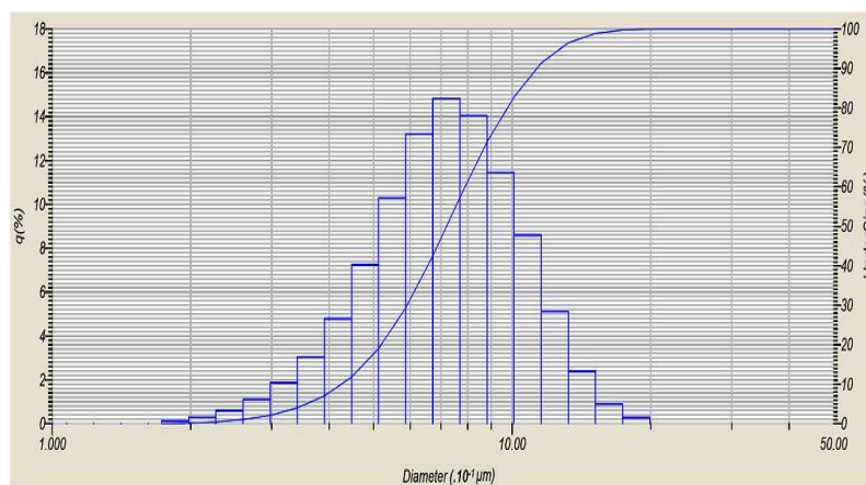
Hình 6. Phân bố kích thước hạt của mẫu HY3 xác định bằng phổ tán xạ laser
