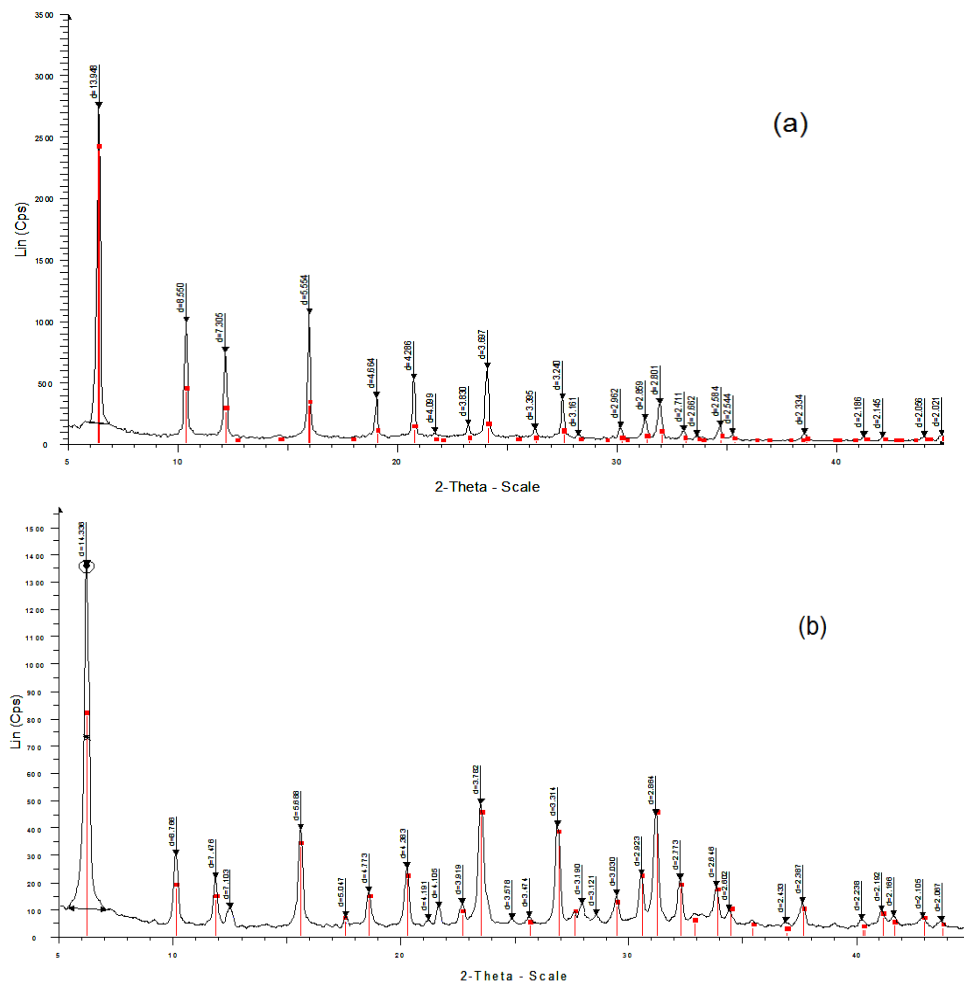
Hình 5. Phổ XRD của hai mẫu (a): NaY3 và (b): NaY1 tương ứng với thời gian già hóa là 12 giờ và 24 giờ
