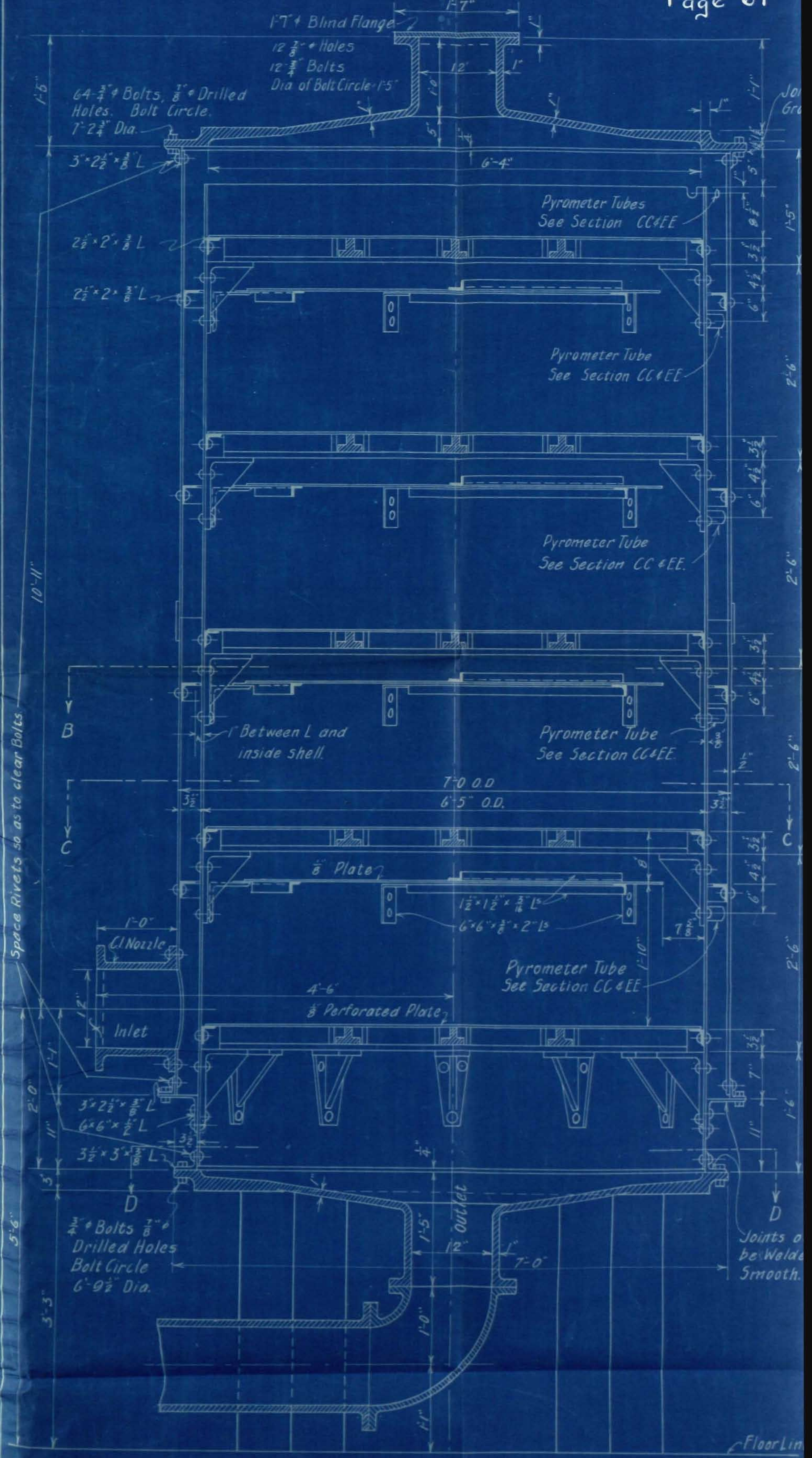
Section A.A
