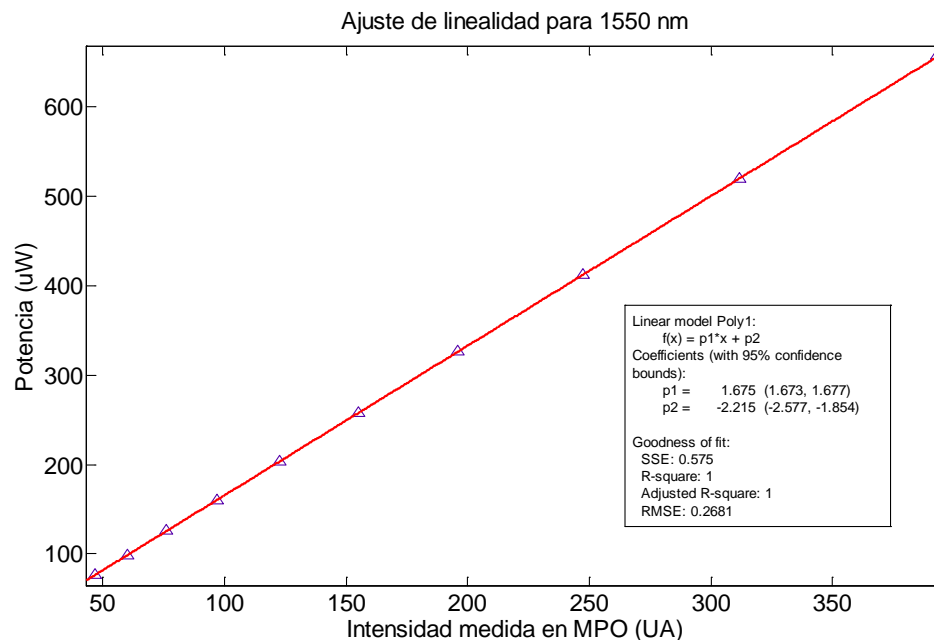
Fig. 4. Función lineal de ajuste de potencia del MPO para 1 550 nm.
