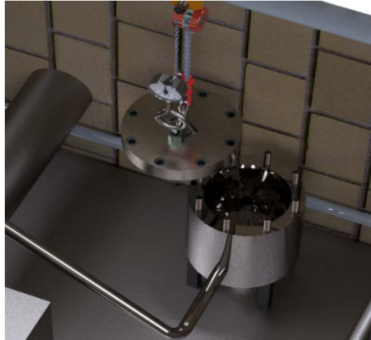
Figura 2 Reactor de explosión súbita de vapor.
