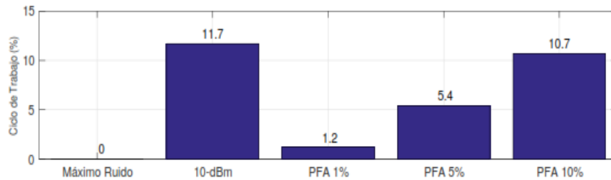
Figura 5 Ciclo de Trabajo en banda con baja ocupación espectral (2.9-3 GHz).
