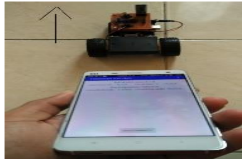
Gambar 11 Robot bergerak maju
