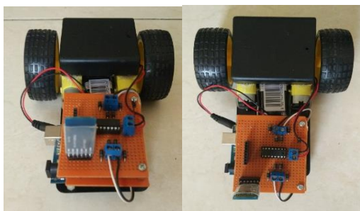
Gambar 10 Tampilan dari robot beroda
