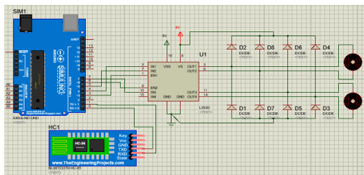
Gambar 4 Rangkaian schematic robot beroda
