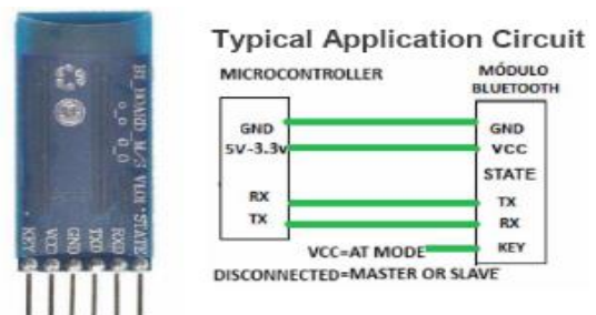
Gambar 3 Konfigurasi pin out dari HC-05.
