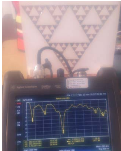
Figura 8 Analizador de cables y antenas midiendo el coeficiente de reflexión.
