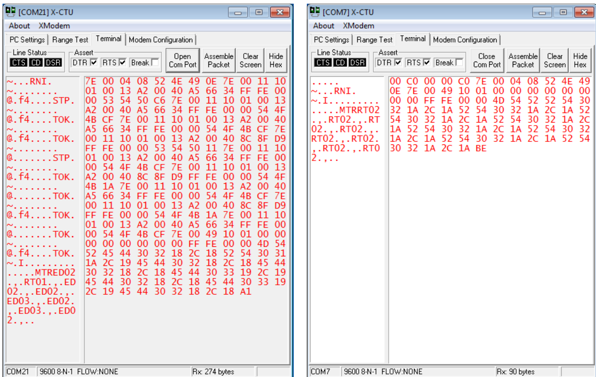
(a) (b) Fig. 6. Comparación de nodos R con y sin hijos.
