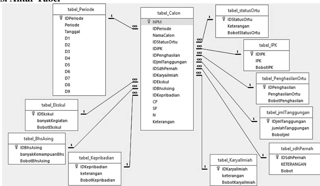
Gambar 3. Relasi Tabel
