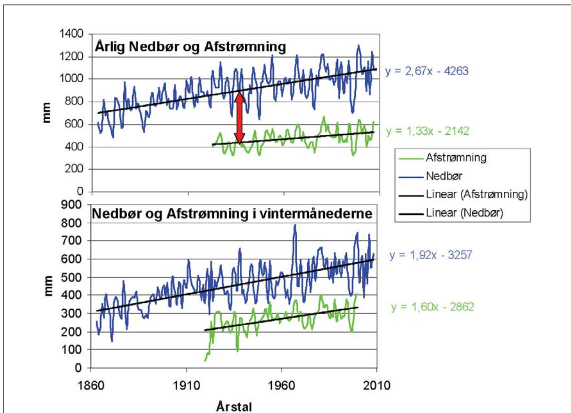
Figur 4. Nedbør og afstrømning fra Alergårde målestation; den røde pil markerer forskellen der skyldes fordampningen. Nederst – Det samme plot men kun for vintermånederne oktober, november, december, januar, februar og marts.
