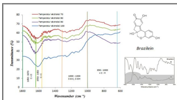
Gambar 3.1 Spektrofotometer infra merah ZWA merahsecang
