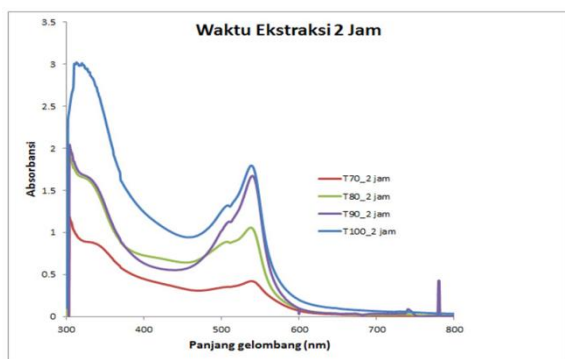
Gambar 3.3. Spektrum UV Vis ZWA merah secang dengan variasi temperatur.
