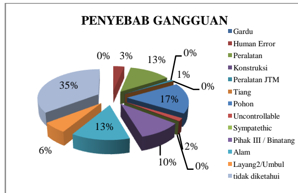
Gambar 5. Grafik Penyebab Gangguan Penyulang GI Industri Tahun 2017
