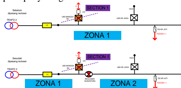
Gambar 7. Single Line Diagram Pemasangan Recloser pada Jaringan Distribusi Penyulang Industri 5 (I.5)
