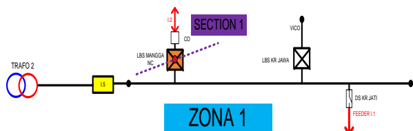
Gambar 3. Pembagian Zona, dan Section
