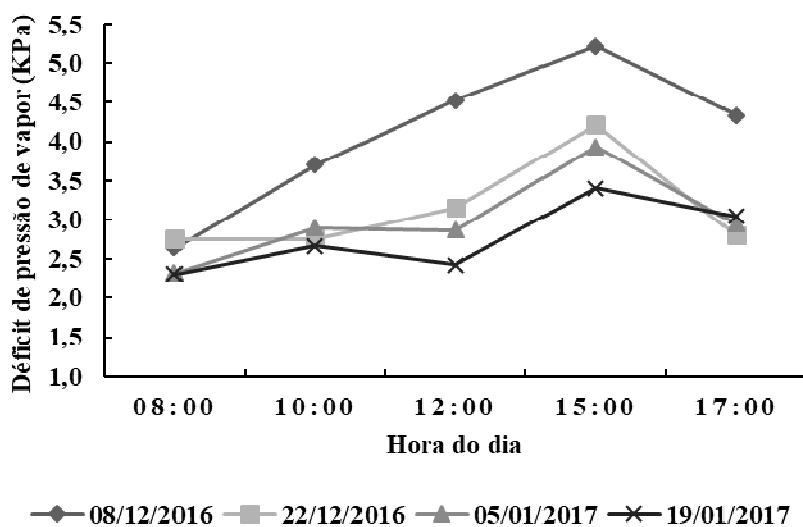
Figura 1. Avaliações quinzenais de déficit de pressão de vapor (KPa), ao longo do dia das plântulas de Myracrodruon urundeuva Allemão.
