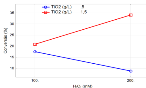
Figura 4 – Médias marginais de conversão de DQO.
