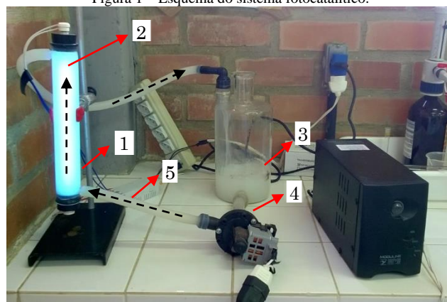
Figura 1 – Esquema do sistema fotocatalítico.
