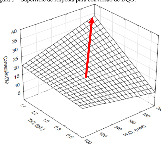
Figura 3 – Superfície de resposta para conversão de DQO.
