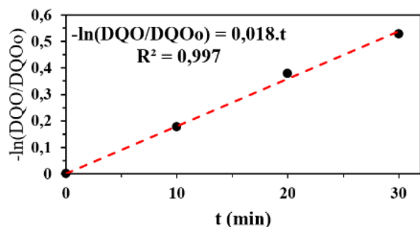
Figura 6 – Cinética de primeira ordem para 1,5 g/L de TiO_2 e 200 mM de H_2O_2 .
