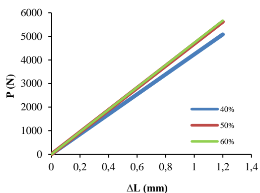
Gambar 1. Grafik hubungan antara Beban P (N) terhadap Pertambahan Panjang \Delta L (mm)
