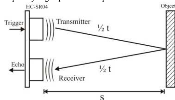
Gambar 2. Prinsip kerja sensor ultrasonik
