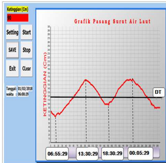
Gambar 5. Hasil pengukuran pasang surut air laut
