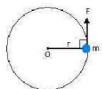
Gambar 2.4 sebuah partikel berotasi mengelilingi sumbu yang berpusat titik 0 Sumber: Sutrisno. 1984. “ Fisika Dasar 2 Mekanika
