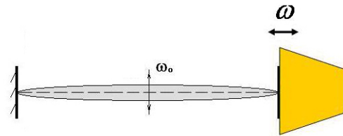
Abb.7: Schematische Darstellung des Melde-Experiments mit einem Bass-Lautsprecher anstelle der Stimmgabel .
