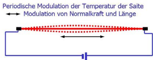
Abb.3: Die so hervorgerufenen Temperaturos zillationen bewirken eine Modulation der thermischen Ausdehnung, in deren Folge auch die Normalkraft variiert, mit der die Saite eingespannt wird (angedeutet durch den schwarzen Pfeil).
