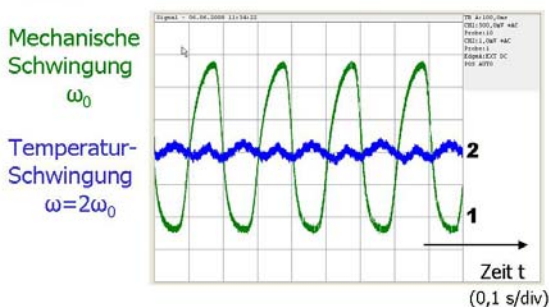
Abb.4: Auslenkung und Temperatur des Drahtes. 1: A_{mech} (2mm/div) 2: A_{Temp} (5°C/div)
