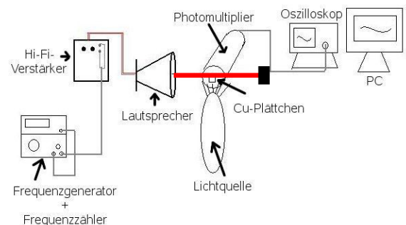
Abb.8: Photos und Skizze des Versuchsaufbaus zur Untersuchung der parametrischen Schwingungen (modifiziertes Melde-Experiment).
