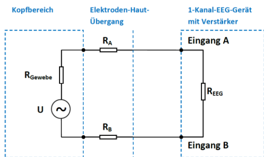
Abb. 6: Einfaches Ersatzschaltbild des Eingangsbereichs eines 1-Kanal-EEG-Geräts [5]; die Potentialschwankungen im Kortex werden durch eine Wechselspannungsquelle sowie organische Gewebestrukturen und zentrale Bauteile des EEG-Geräts durch ohmsche Widerstände elementarisiert.
