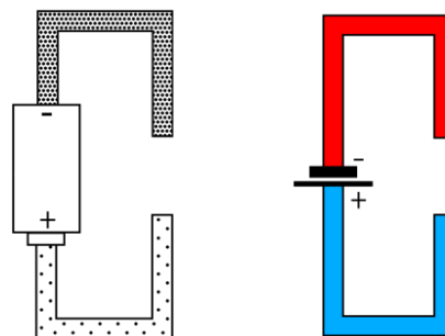
Abb.3: Punktgedichtdarstellung (links) und Farbdarstellung (rechts) des elektrischen Drucks
