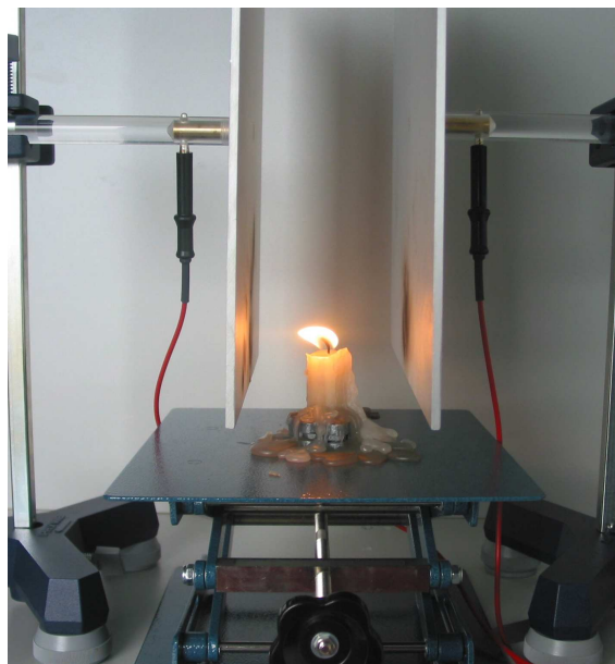
Abb.11: Kerze in einem Plattenkondensator
