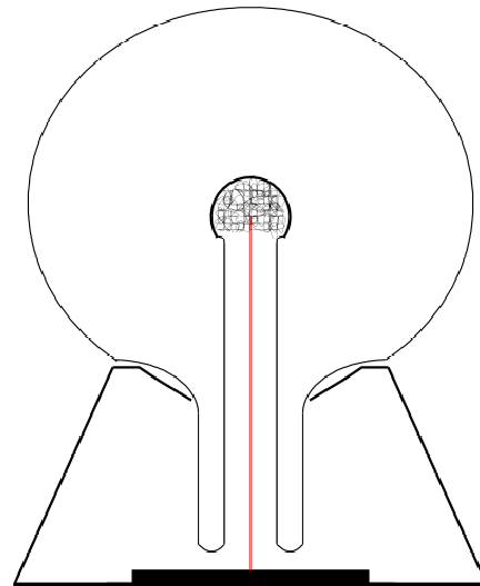
Abb.7: Schematische Darstellung einer Plasmakugel
