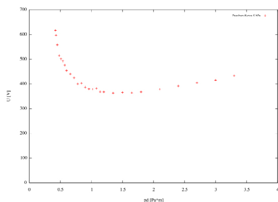
Abb.2: Paschen-Kurve für Luft bei einem Druck von 6 hPa
