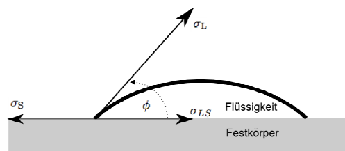
Abb.4: Zusammenhang zwischen Oberflächenenergien und Kontaktwinkel
