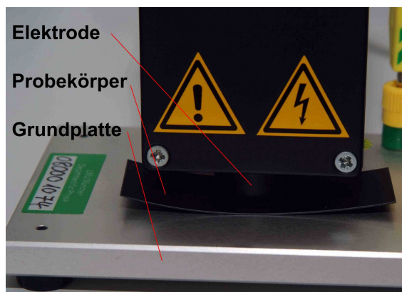
Abb.3: Elektrode zur Behandlung eines Probekörpers
