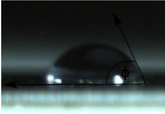
Abb.5: Aufnahme eines Tropfens in Seitenansicht
