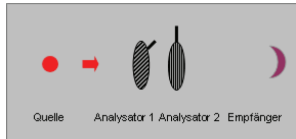
Abb. 3: Transmission eines Photons durch zwei Polarisationsfilter
