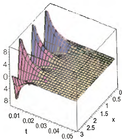
Fig. 2. Comportamiento gráfico de la Ec.(5), referente a la solución del problema con y. 0 \leq x \leq 3,0
