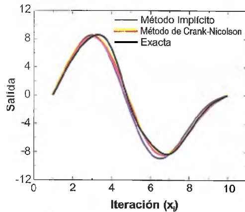
Fig. 4. Gráfico que muestra el comportamiento de la solución numérica con la exacta dada por la Ec.(5), obtenidas tanto por el MI, como por el MCN, para la situación en que, t_{\max} = 0,0010s , manteniendo k y a_n constantes.
