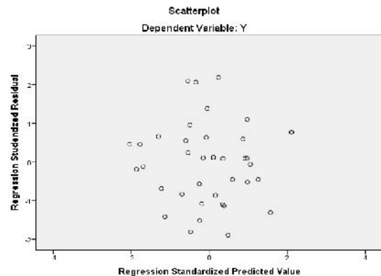
Gambar 1. Grafik Scatterplot
