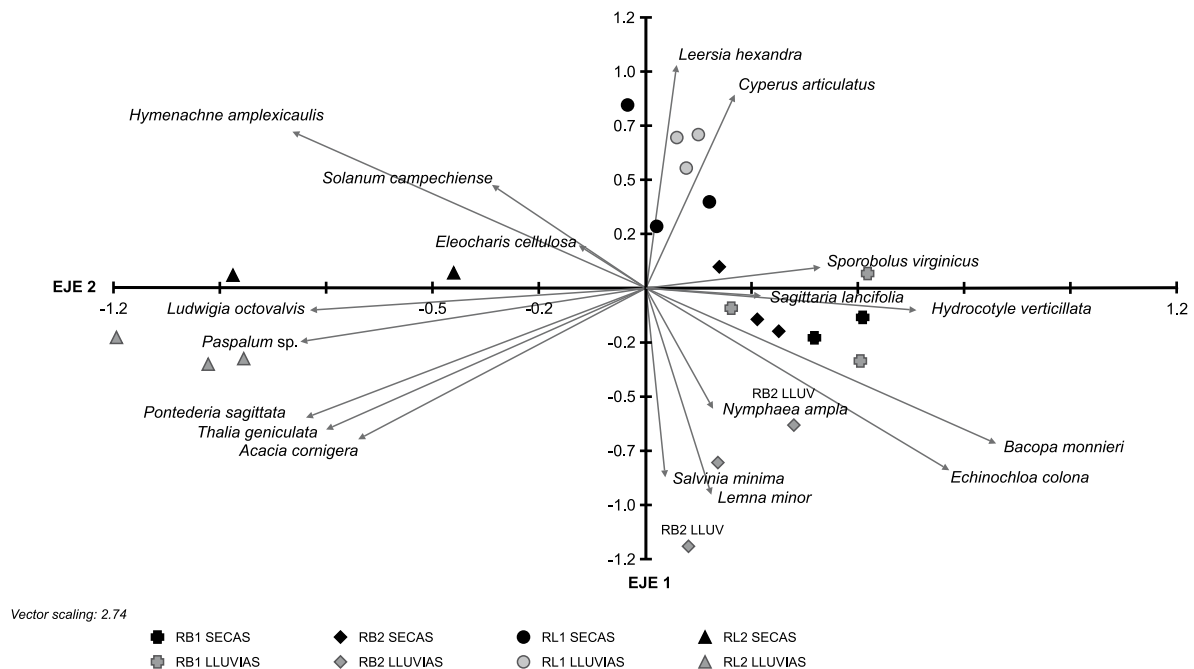
Figura 2: Asociación de las cuatro localidades de estudio (casos) con 18 especies (variables) con respecto a los dos componentes principales. Los dos componentes principales explican 46% de la variación. Sobre el primer componente se establece un gradiente de intensidad de forrajeo con los sitios de mayor intensidad en el extremo izquierdo (RL2). Dentro de cada sitio las épocas del año tienden a separarse sobre el eje dos en función de la temporalidad de secas-lluvias, excepto para el sitio RL1.
