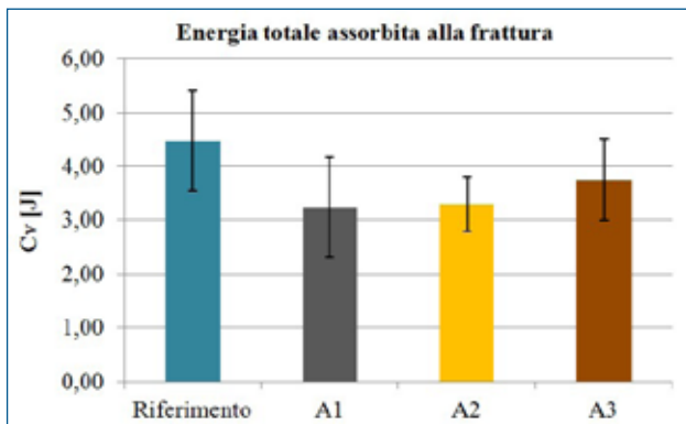
Fig. 7 – Confronto tra le energie totali all’impatto misurate dal pendolo per la lega A356 trattata con gli affinanti A1, A2 e A3, rispetto al Riferimento. La deviazione standard è riportata come barra di errore.
