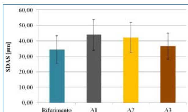
Fig. 3 – Confronto tra le dimensioni medie dello SDAS per la lega A356 trattata con gli affinanenti A1, A2 e A3, rispetto al Riferimento. La deviazione standard è riportata come barra di errore.
