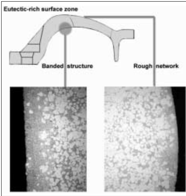
Fig. 6b – Thixoformed AlSiMg 0.6 T5 alloy disc.
