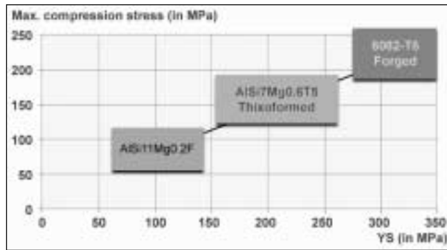
Fig. 12 – Relazione fra massimo carico di compressione e carico di snervamento.
