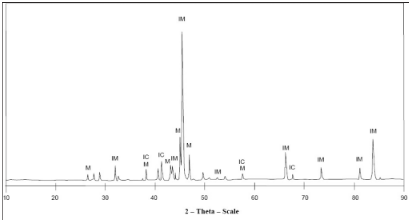
Fig. 7 – XRD of ferromanganese alloy produced from the smelting of manganese ore sinter fines cold bonded with 9% cement addition. Fig. 7 – XRD di una lega di ferromanganese prodotta mediante smelting di manganese ore sinter fines legate a freddo con aggiunta di cemento al 9%.
