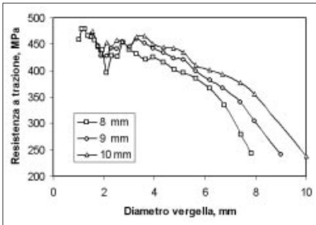
Fig. 7 – Variazione della resistenza alla trazione per effetto della trafilatura in vergelle con diametro iniziale diverso.
