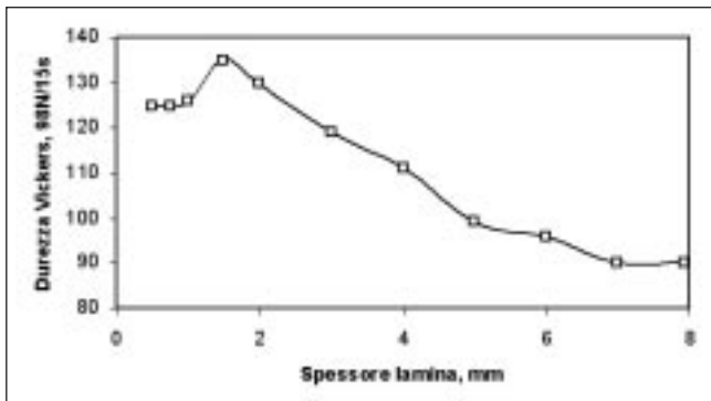
Fig. 8 – Variazioni di durezza Vickers per effetto della laminazione.
