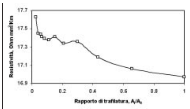
Fig. 5 – Variazione della resistività elettrica per effetto della trafilatura.
