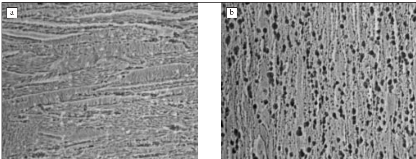
Fig. 12 – Microstruttura di una lamina di spessore 1 mm: sezione longitudinale (a) e trasversale (b).
