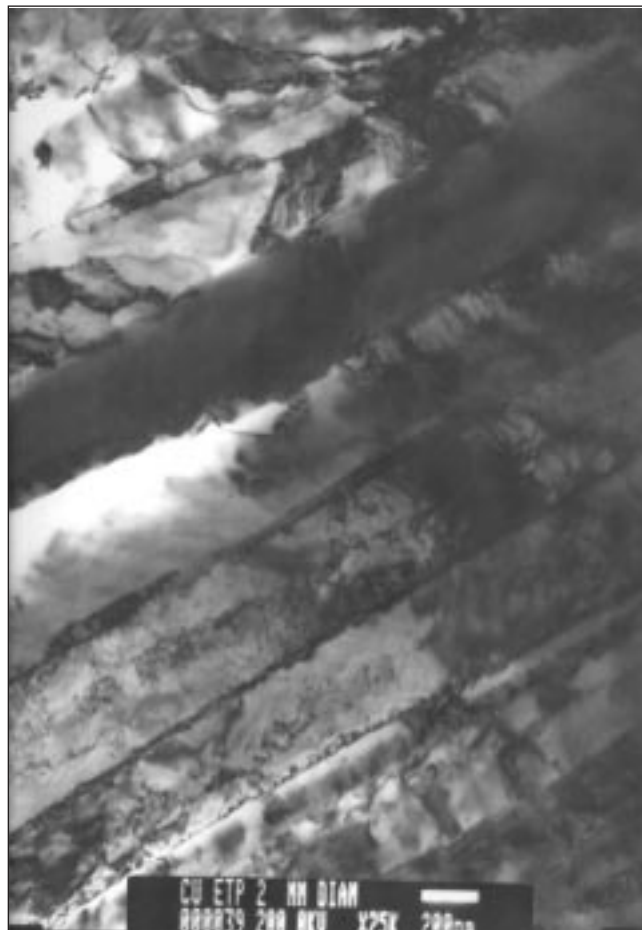
Fig. 1 – Microstruttura della sezione longitudinale del filo di Ø 2 mm: grani allungati nella direzione della trafilatura.
