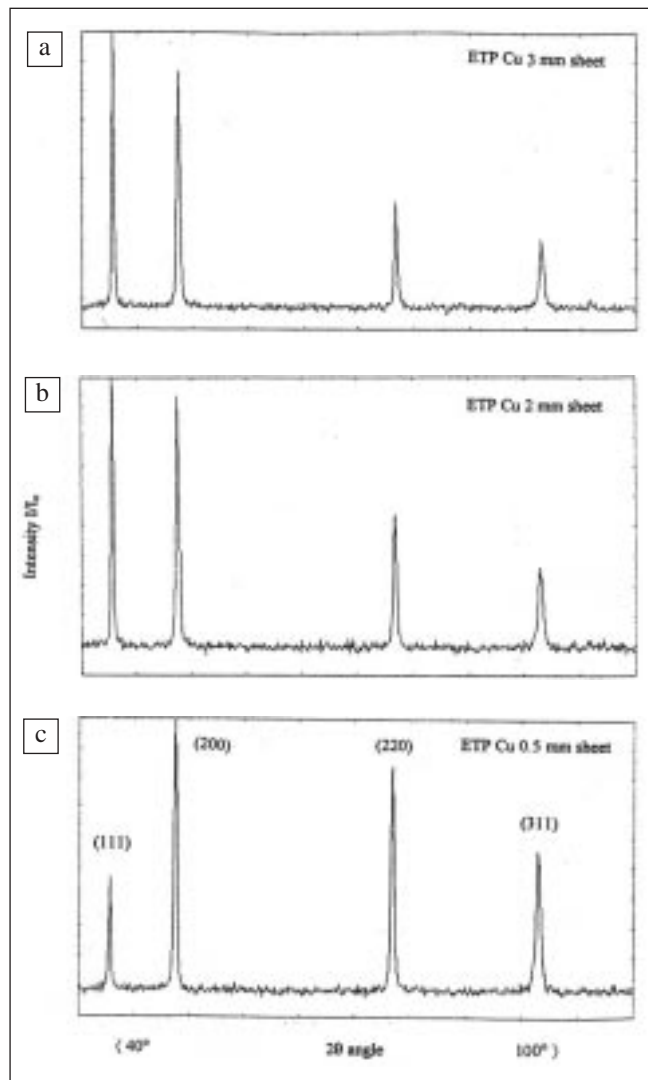
Fig. 14 – Attivazione di diversi piani di scorrimento durante la laminazione: diffrattogrammi delle lamine di spessore 3 mm (a), 2 mm (b) e 0.5 mm (c).
