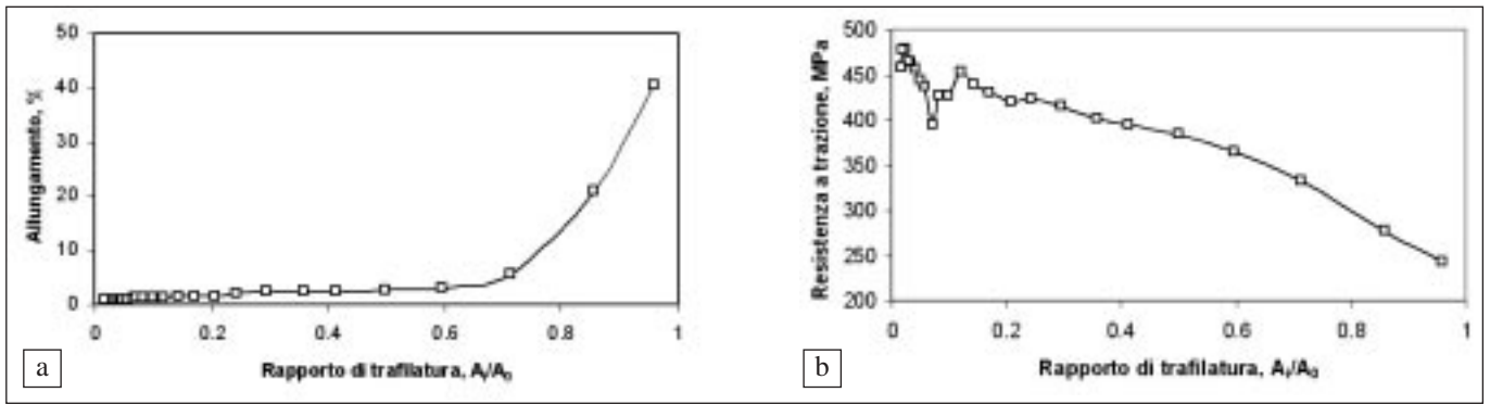
Fig. 6 – Variazione dell’allungamento (a) e della resistenza alla trazione (b) per effetto della trafilatura.
