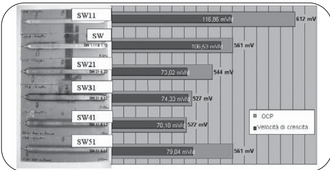
Fig. 8 Potenziale di libera corrosione finale e velocità del potenziale dei campioni saldati esaminati in acqua di fiume sintetica in presenza di batterie ossidanti del manganese. Final reached corrosion potential and increasing rate of the examined stainless steels in synthetic river water in the presence of manganese oxidising bacteria.
