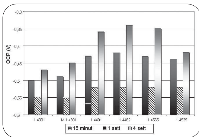
Fig. 12 Potenziale di libera corrosione degli acciai esaminati nell'acqua dell'impianto di trattamento delle acque. Free corrosion potential of the examined stainless steels in the water treatment plant.
