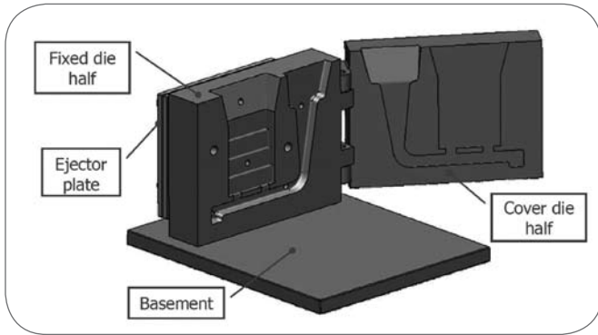
▲ Fig. 1 Permanent mould die used in the present work. Stampo permanente in acciaio utilizzato in questo studio.
