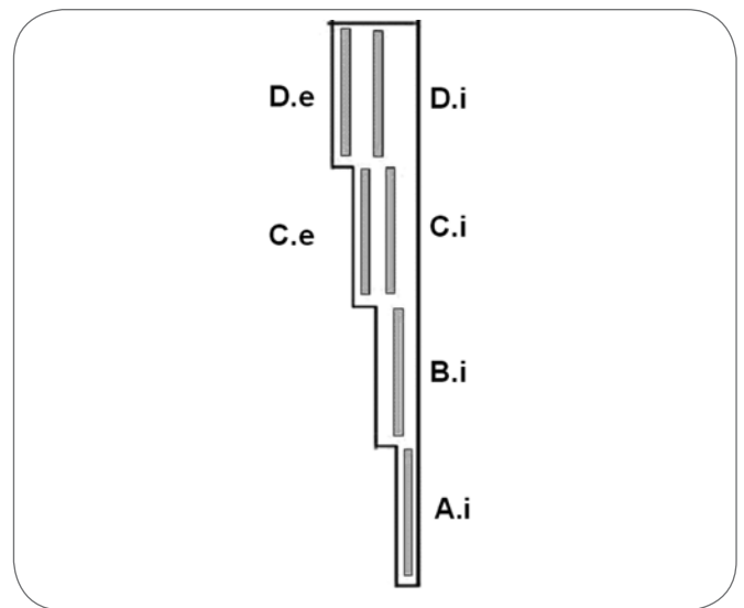
▲ Fig. 3 Side view of the step casting showing sectioning scheme. Vista laterale del getto con evidenziate le zone di prelievo dei campioni per l'analisi microstrutturale e delle proprietà meccaniche.
