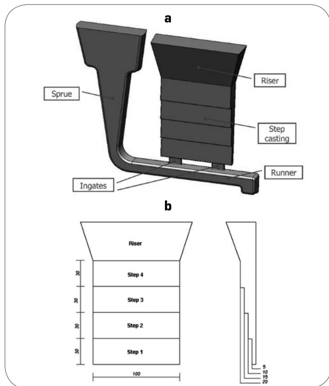
▲ Fig. 2 (a) The step casting CAD geometry with (b) front and side views. All the measures are in mm. (a) Geometria CAD e (b) vista frontale e laterale del getto a gradini, utilizzato in questo studio. Tutte le misure sono espresse in mm.
