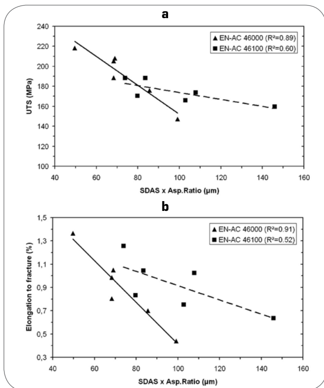
Fig. 8 Average (a) UTS and (b) elongation to fracture as a function of the combined parameter SDAS x Aspect ratio; coefficient of determination, R2, are given. Data refer to EN-AC 46000 and 46100 alloys. Valori medi di (a) UTS e (b) allungamento a rottura in funzione del prodotto tra SDAS e rapporto d'aspetto. E' inoltre riportato in coefficiente di determinazione, R2. I dati si riferiscono alle leghe EN-AC 46000 e EN-AC 46100.
