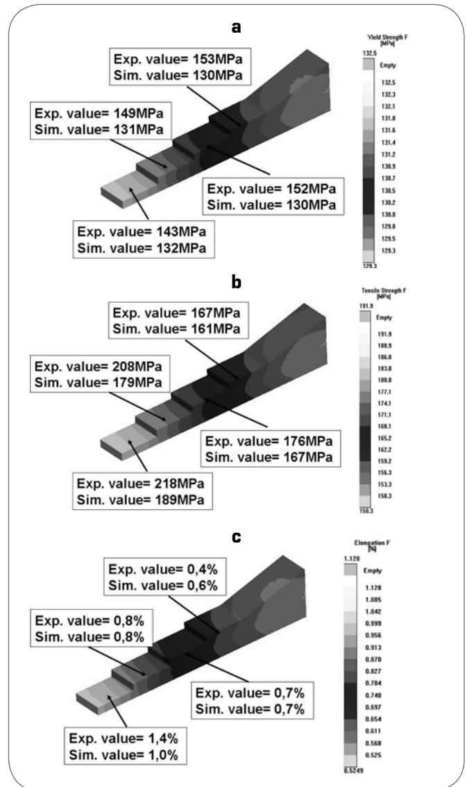
Fig. 9 Comparison between experimental and simulated mechanical properties in EN-AC 46000 step casting. The images refer to (a) YS, (b) UTS and (c) elongation to fracture. Confronto tra i valori delle proprietà meccaniche ottenuti sperimentalmente e mediante simulazione di processo per il getto colato con lega EN-AC 46000. Le immagini si riferiscono a (a) YS, (b) UTS e (c) allungamento a rottura.
