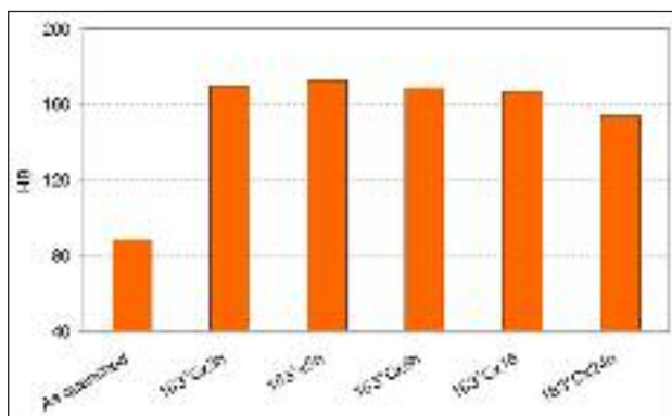
FIG. 1 Hardness values at 163°C. Valori di durezza a 163°C.
