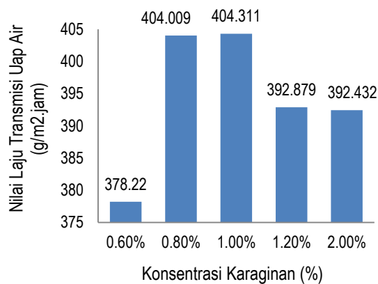
Gambar 5. Pengaruh konsentrasi terhadap nilai laju transmisi uap air bioplastik
