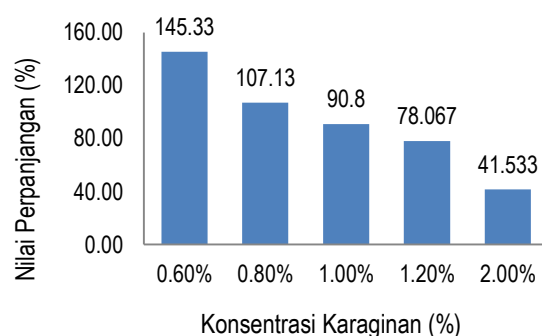
Gambar 4. Pengaruh konsentrasi karaginan terhadap nilai perpanjangan bioplastik
