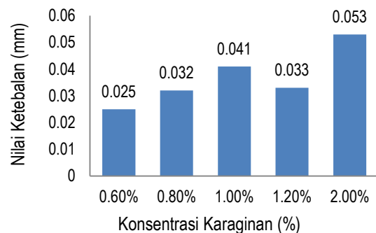
Gambar 1. Pengaruh konsentrasi karaginan terhadap ketebalan bioplastik
