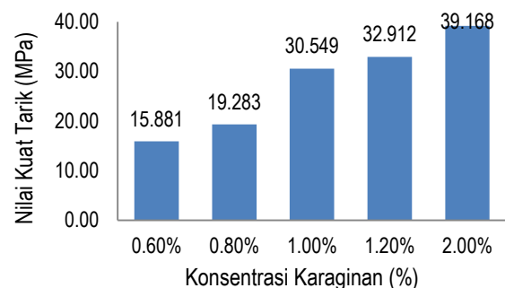
Gambar 3. Pengaruh konsentrasi karaginan terhadap kuat tarik bioplastik
