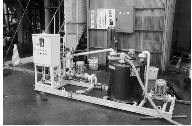
写真2 加水装置
