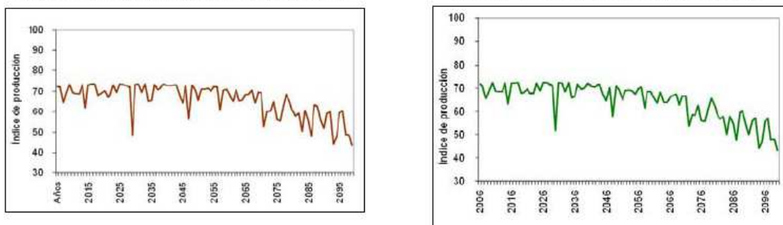
Figura 7. Proyección de los índices de producción agropecuaria y de cultivo para escenario A2.
