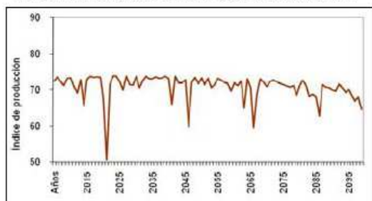
NICARAGUA: PROYECCIONES DEL ÍNDICE DE PRODUCCIÓN AGROPECUARIA A PARTIR DEL ESCENARIO B2
