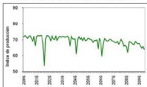
NICARAGUA: PROYECCIONES DEL ÍNDICE DE PRODUCCIÓN AGRÍCOLA A PARTIR DEL ESCENARIO B2
