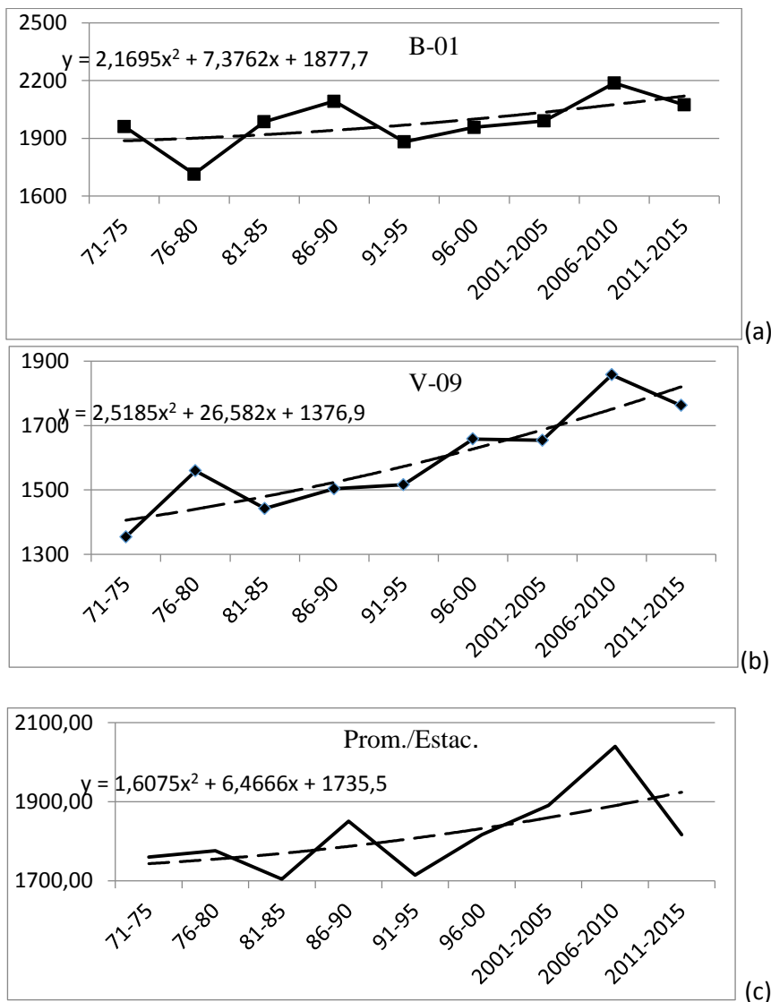
Fig. 11 Acumulados promedios anuales (mm) por lustro para las Estaciones que se muestran (a y b) y para el conjunto de las 8 Estaciones (c). Las líneas de ajustes polinomiales se representan por líneas de guiones y cuyas ecuaciones aparecen en la parte superior de cada gráfico.
