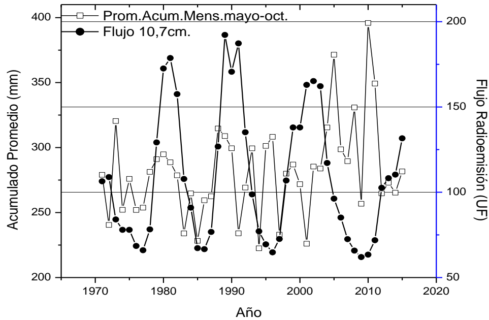
Fig. 9 Comparación de valores anuales del Flujo de Radioemisión Solar y el acumulado promedio anual de precipitación para toda la muestra. La línea con círculos negros corresponde al Flujo Solar y la de cuadrados sin relleno al Promedio Acumulado. (1 UF = 10^{-22} \text{ W/m}^2 \cdot \text{Hz}^{-1} ).
