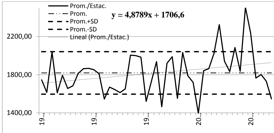
Figura 4. Promedios anuales del acumulado por estación (mm.)
