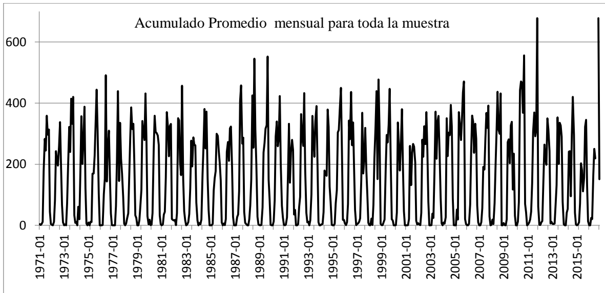
Fig. 3 Serie de tiempo de 45 años de los acumulados mensuales (mm) promedio de las 8 Estaciones
