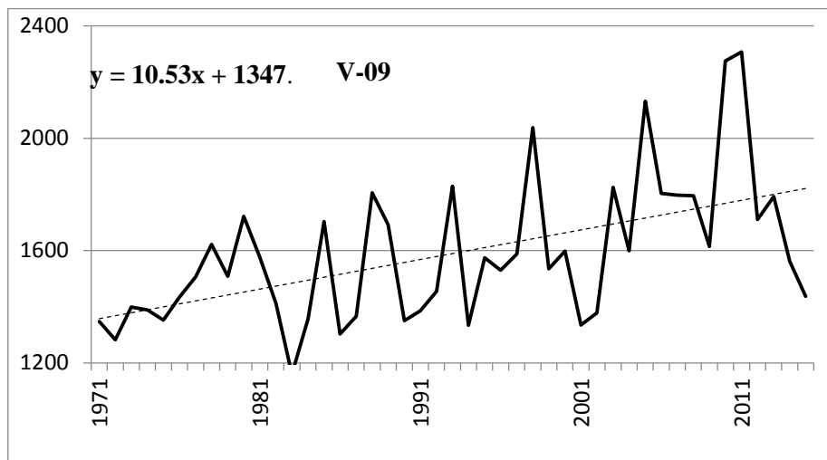
Fig. 5 Acumulados anuales (mm.) de la Estación V-09. La línea punteada representa la tendencia lineal ajustada cuya ecuación se muestra en la esquina superior izquierda.
