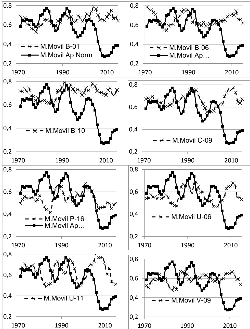
Fig. 8 Relación temporal entre los promedios anuales (normalizados y suavizados) del índice geomagnético Ap y los acumulados de lluvia de los meses de agosto + septiembre (normalizados y suavizados) para las 8 estaciones utilizadas.
