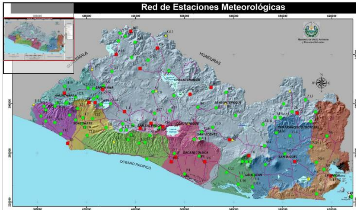
Fig. 1 Red de Estaciones Meteorológicas de El Salvador (Fuente; http://www.snet.gob.sv , Servicio Nacional de Estudios Territoriales).
