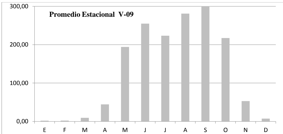
Fig. 6 Muestra del comportamiento estacional del promedio acumulado mensual (mm), en este caso para la V-09, las demás son muy semejantes. El resultado se obtiene de la superposición de los 45 años observados.
